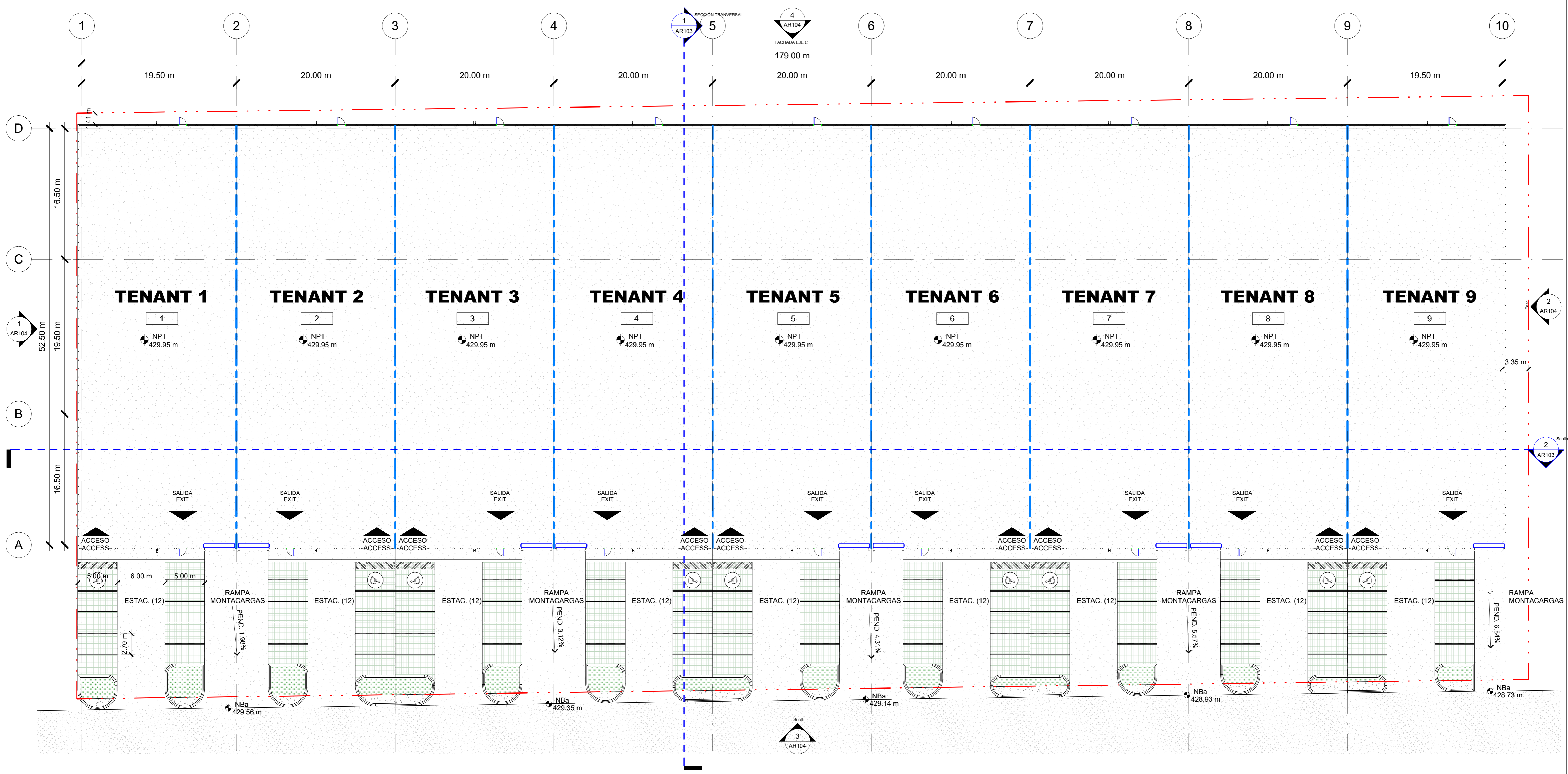
1 PLANTA ARQUITECTÓNICA GENERAL AR103 ESC 1 : 250
